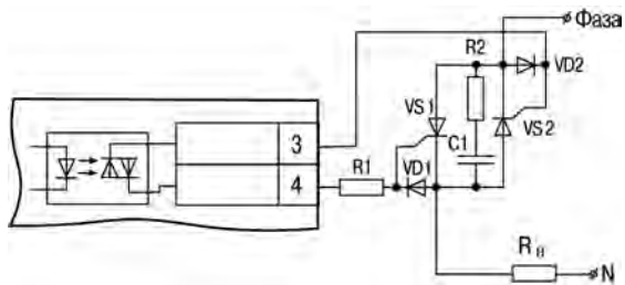
Рисунок 5.8 – Схема подключения двух встречно-параллельно включенных тиристорov к ВУ типа С
